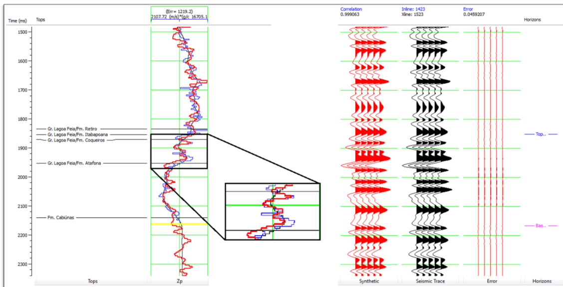
Figura 33: Janela de análise da inversão em um dos poços no Hampson-Russel com destaque para o intervalo da Formação Coqueiros.
