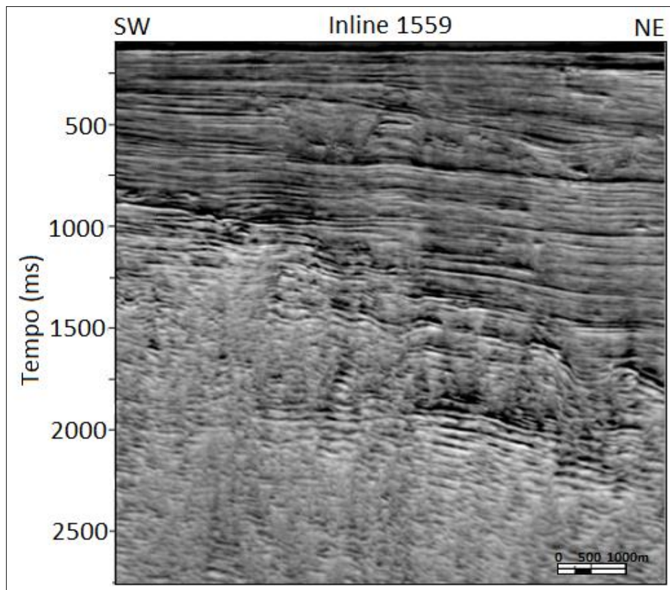
Figura 29: Atributo TecVA aplicado em uma seção sísmica.
