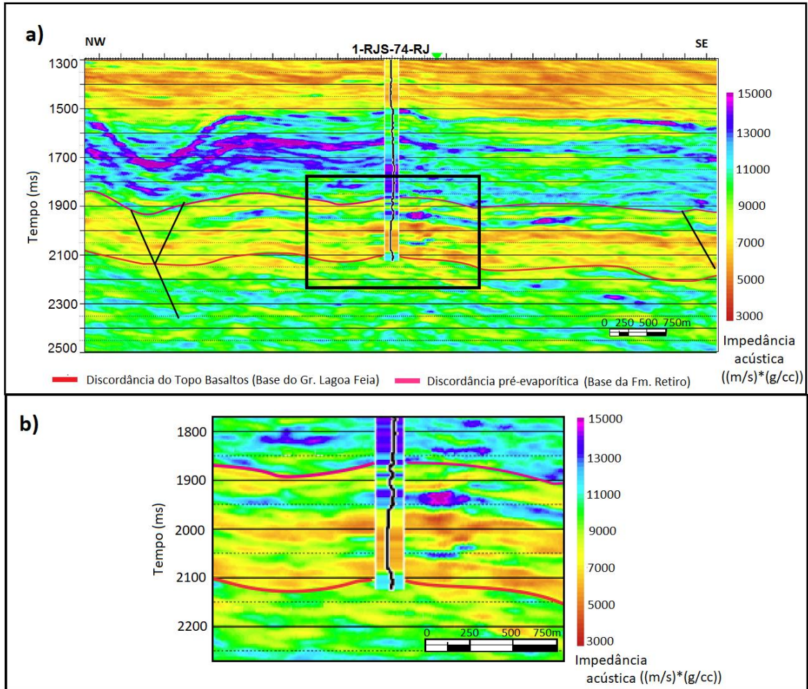
Figura 40: Resultado da inversão model-based na crossline 1438 e no poço 1-RJS-74-RJ. Destaque para a impedância obtida no poço cego; (b) Zoom da imagem a, para dar destaque a região do poço.
