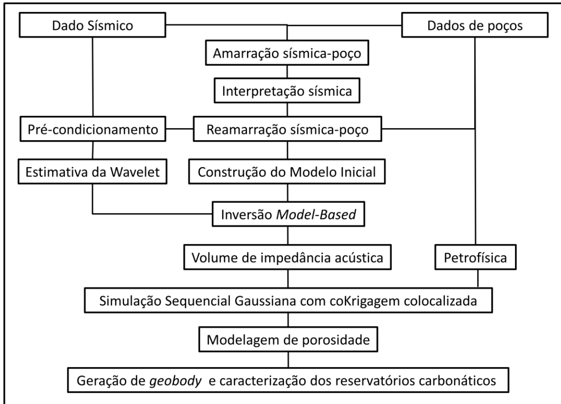
Figura 28: Fluxo de trabalho utilizado na caracterização dos reservatórios carbonáticos aptianos do Campo de Linguado.
