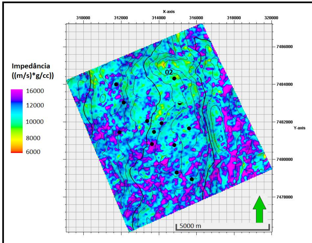
Figura 44: Mapa com os valores de impedância acústica sobre o topo do Grupo Lagoa Feia, base da sequência evaporítica.
