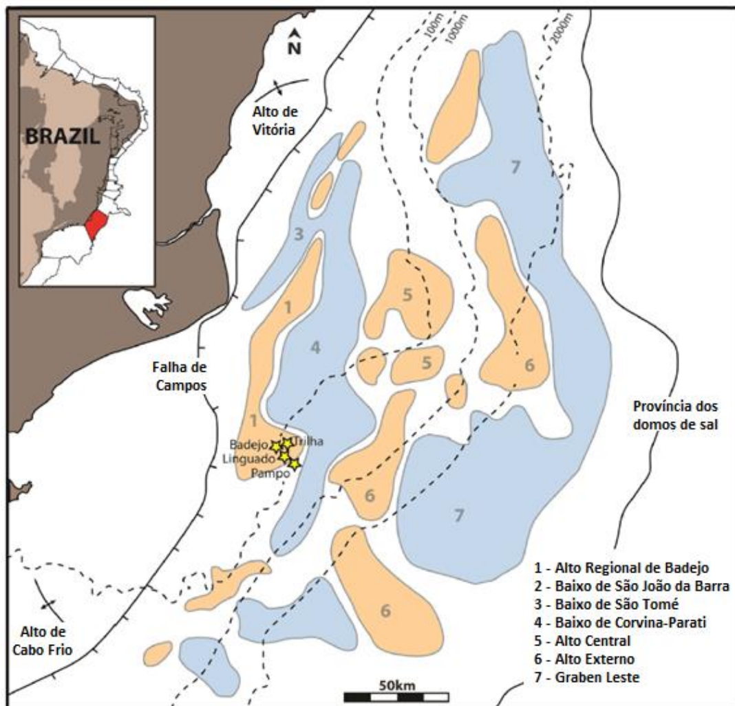
Figura 7: Mapa estrutural da Bacia de Campos. Principais altos (em laranja) e baixos (em azul) estruturais da bacia e localização dos campos produtores de óleo em coquinas (estrelas amarelas). Adaptado de Guardado et al. , 2000.
