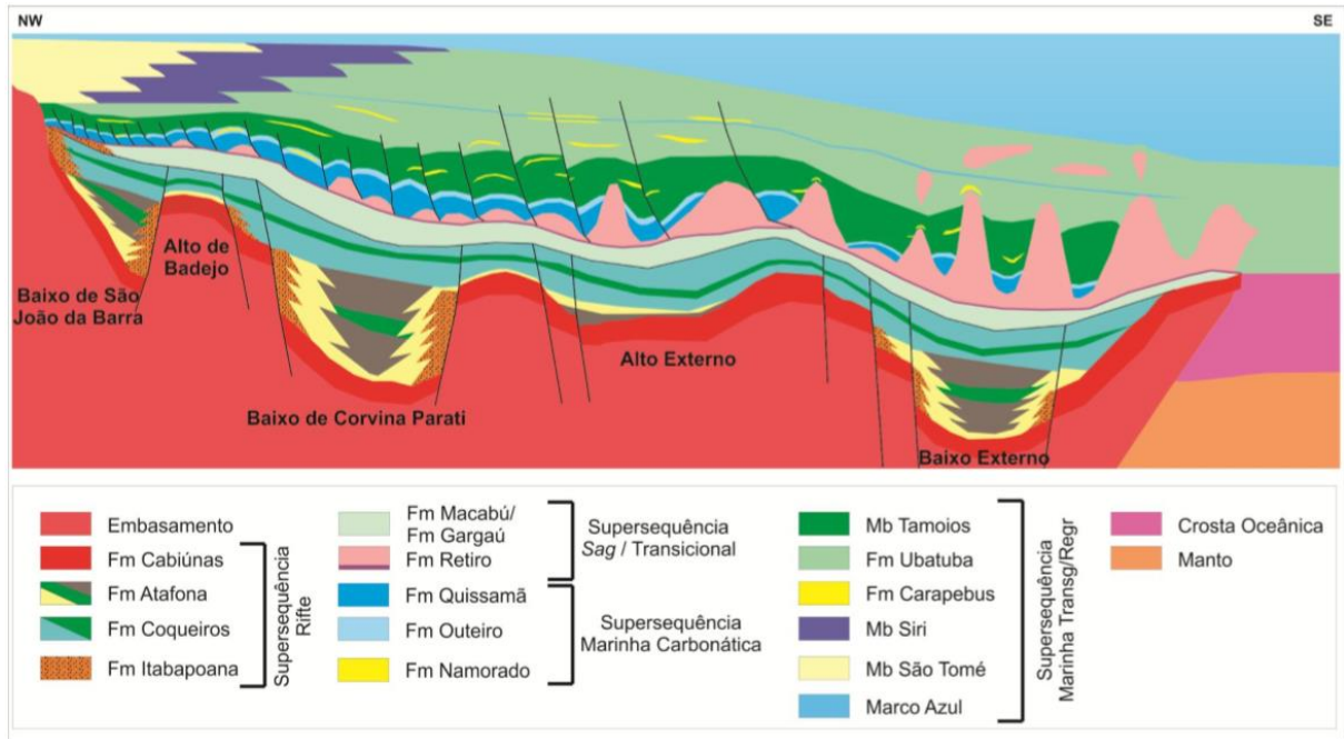
Figura 2: Seção geológica da Bacia de Campos mostrando as supersequências sedimentares depositadas nas fases rifte, pós-rifte (transicional) e drifte. Fonte: Rangel et al. , (1998).
