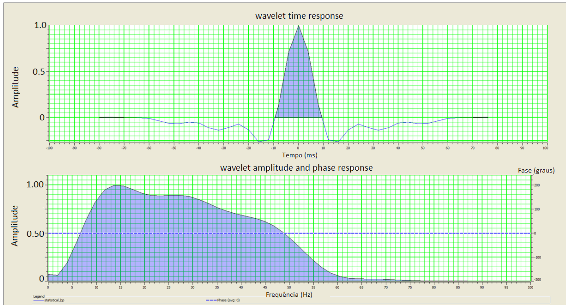
Figura 31: Wavelet extraída a partir do espectro de amplitude do volume sísmico pré-condicionado.
