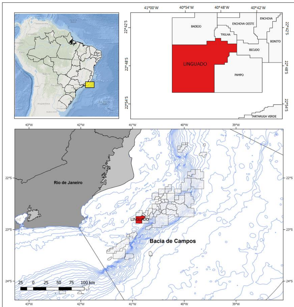
Figura 4: Localização do Campo de Linguado, Bacia de Campos.
