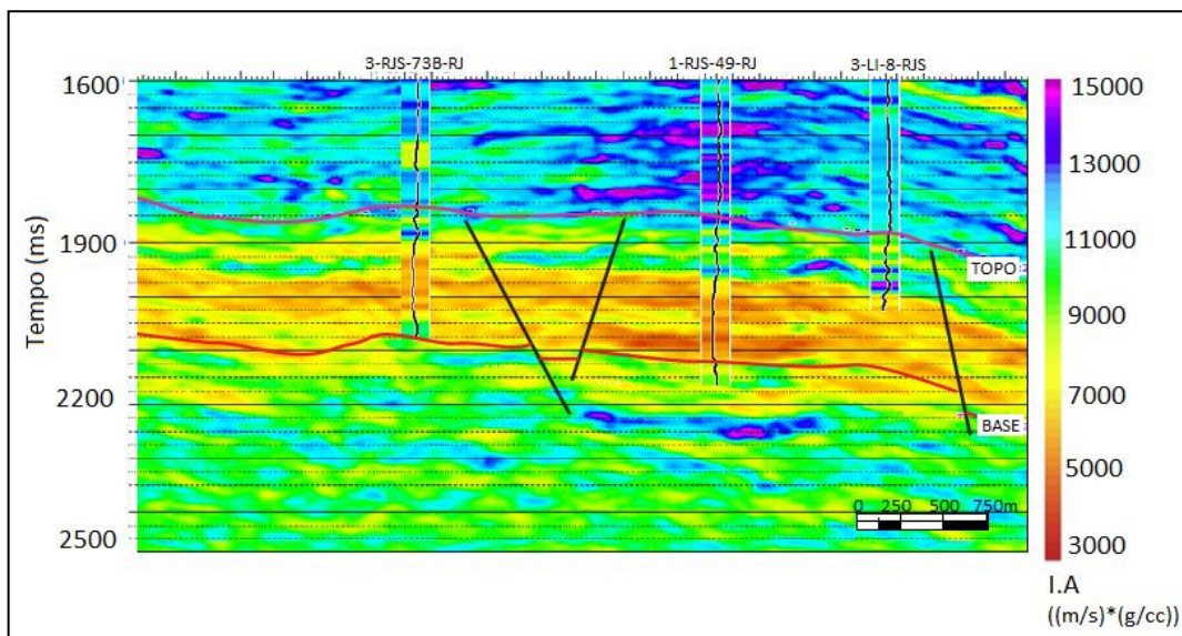
Figura 41: Linha arbitrária AB1 com os valores de impedância acústica, passando pelos poços 3-RJS-73B-RJ, 1-RJS-49-RJ, 3-LI-8-RJS.
