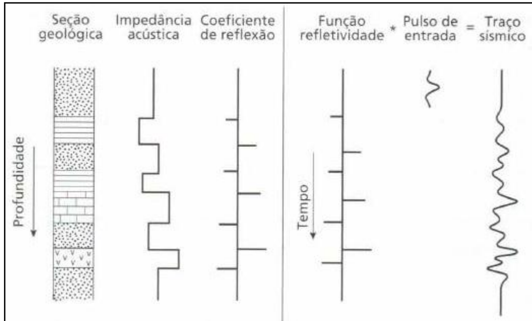
Figura 18: Modelo de convolução do traço sísmico. Esta imagem mostra o traço sísmico como o resultado da função refletividade convolvida com o pulso de entrada, além da relação entre a função refletividade e impedância acústica das camadas geológicas (Kearey et al. , 2002)
