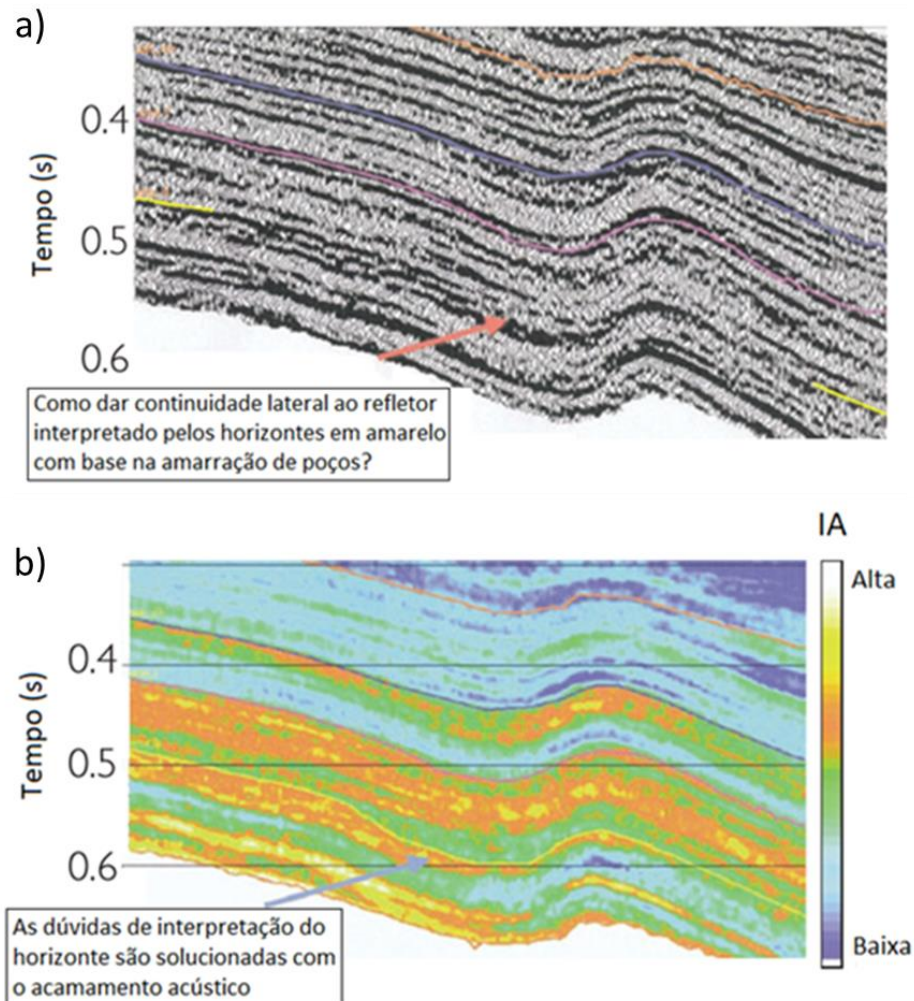
Figura 17: a) Seção sísmica original; b) Seção sísmica invertida para um modelo de impedância acústica (modificado de Latimer et al., 2000).
