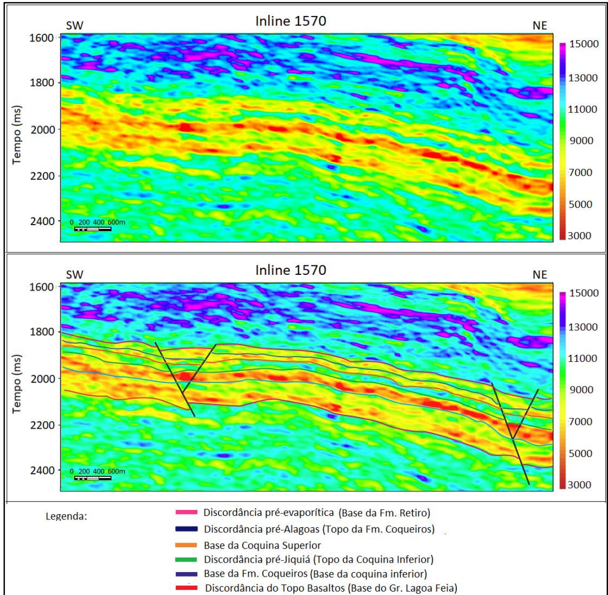
Figura 42: Inline 1570 com resultado da inversão acústica. Os novos horizontes mapeados correspondem a topo e base da coquina inferior e topo e base da coquina superior.
