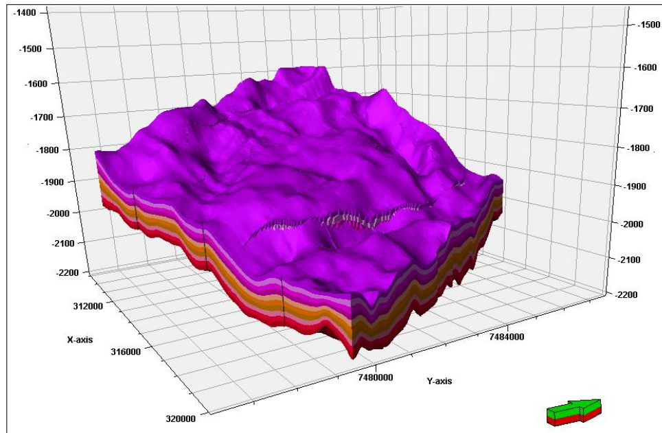
Figura 49: Modelo estrutural contruído entre as superfícies discordância pré-Jiquiá e o discordância pré-avaporítica e falhas mapeadas na seção rift.
