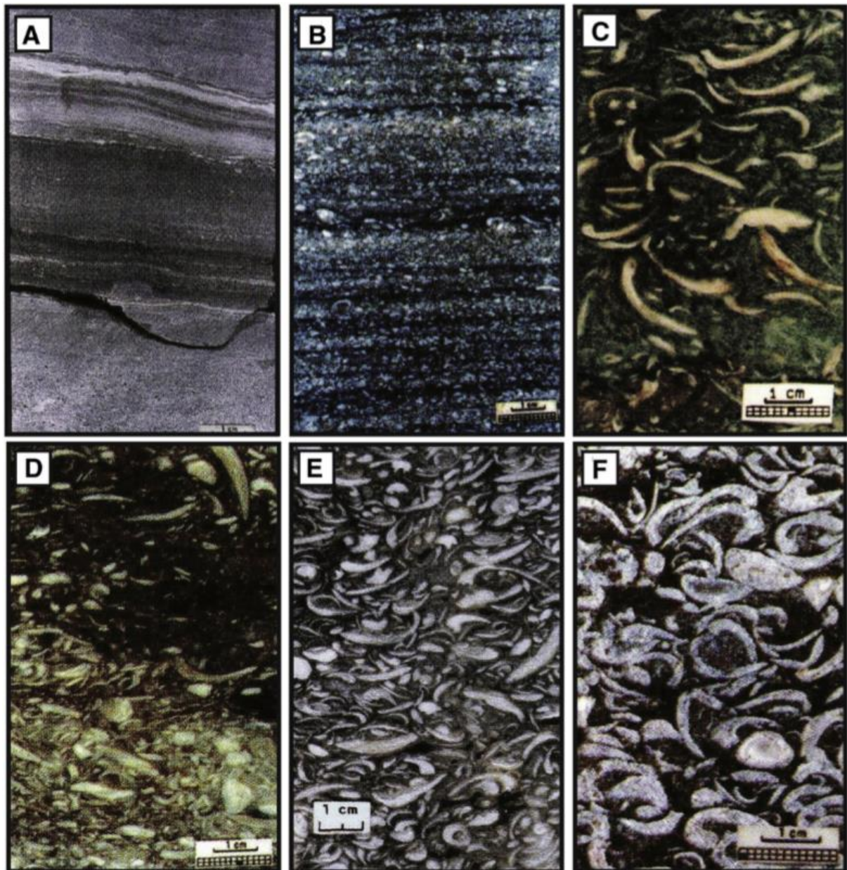
Figura 10: Fotos de amostras de calha de seis associações de fácies de coquinas da Formação Coqueiros. (A) depósitos de margem de lagos, (B) calcarenitos bioclásticos praias, (C) arenitos bioclásticos praias, (D) lençóis bioclásticos bordas de barras, (E) barras bioclásticas; (F) bancos de biocacumulados. (Adaptado de Carvalho et al. , 2000).
