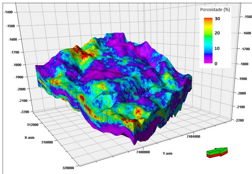
Figura 50: Volume de porosidade da Formação Coqueiros modelado usando o método geoestatístico de Simulação Sequencial Gaussiana com cokrigagem colocalizada.
