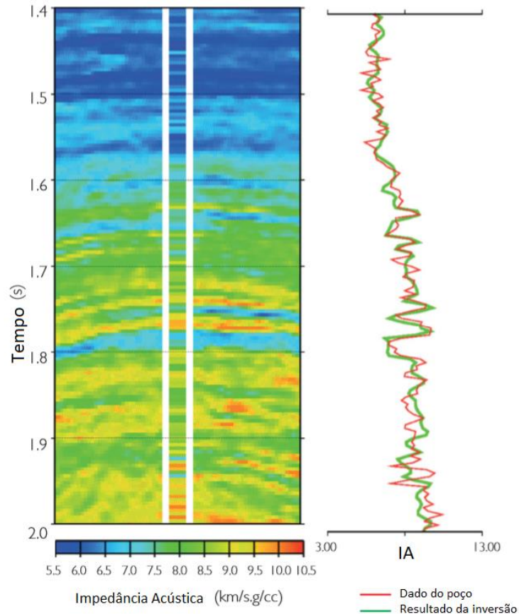
Figura 23: Exemplo de validação da inversão com uso de poço cego. Comparação do resultado da impedância invertida com a impedância calculada a partir dos perfis de poços (after BACH et al. , 2000 em SIMM & BACON, 2014)
