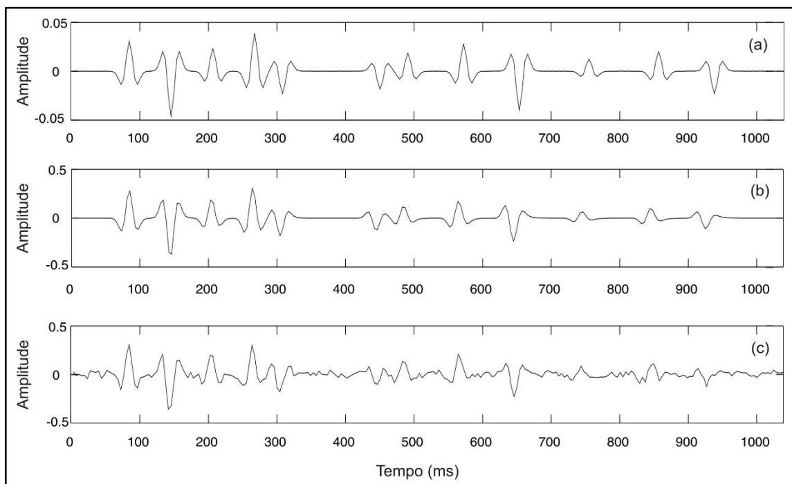
Figura 14: (a) Traço sísmico sintético; (b) traço sísmico sintético com os efeitos de atenuação e dispersão do meio; (c) traço sísmico sintético com ruído randômico e com os efeitos de atenuação e dispersão do meio. Modificado de Lupinacci (2014).
