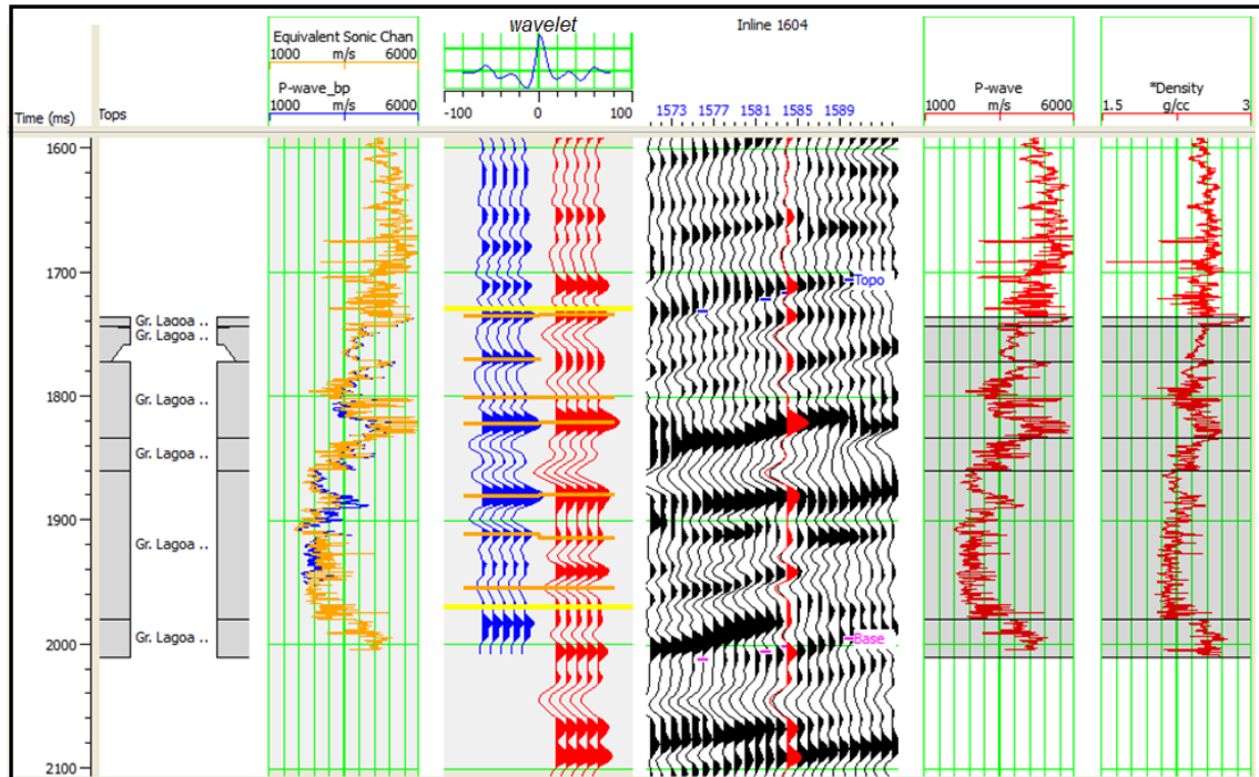
Figura 20: Mostra um processo de amarração poço-sísmica. Os tracks estão organizados da seguinte forma: (1) topos das formações, (2) perfil sônico (curva laranja) e curva de velocidade da onda sísmica compressional (azul) com filtro passa banda de 60 Hz (3) wavelet estimada e traços sísmicos sintéticos (azuis) e reais (vermelhos), (4) seção sísmica mostrando o traço sísmico extraído para a amarração, (5) P-wave, (6) perfil de densidade. (Fonte: A autora)
