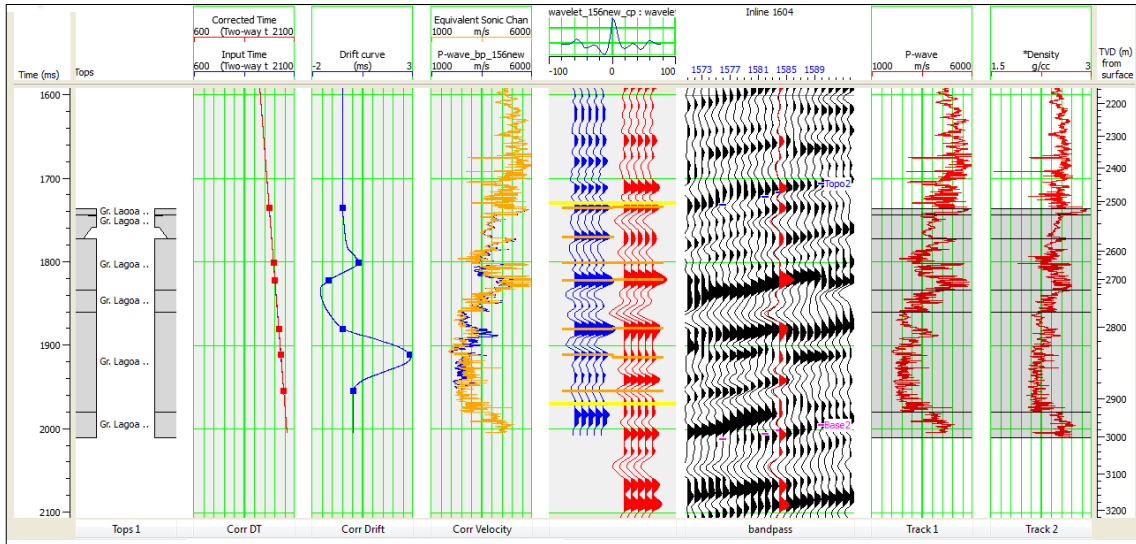
Figura 30: Janela de amarração de um dos poços à sísmica no software Hampson-Russell. Onde cada track corresponde a: intervalo de tempo (1), topo de formações (2), curva de sônico corrigida (3), curva de desvio ( drift ) entre o perfil sônico medido e o sônico calculado (4), amarração do traço sísmico sintético e o traço sísmico original (5), traços sísmicos, local de estimativa do pulso sísmico para amarração em vermelho, e horizontes topo e base interpretados anteriormente (6), perfil sônico medido (7), perfil densidade medido (8), profundidade em metros (9).
