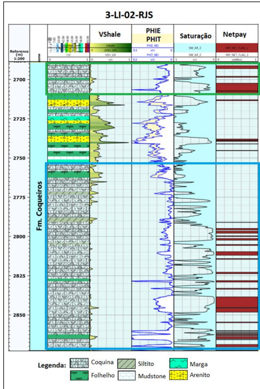
Figura 45: Análise petrofísica no poço 3-LI-2-RJS. Track 1 : Formação Coqueiros; track 2 fácies interpretadas; track 3 : volume de argila (VShale); track 4 : porosidade total (PHIT) e porosidade efetiva (PHIE); track 5 : saturação de água; track 6 : net-pay , Coquina superior: retângulo verde, coquina inferior: retângulo azul.
