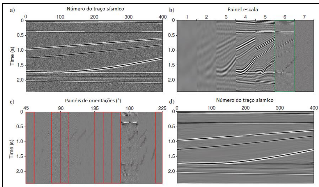
Figura 13: Fluxo de trabalho da filtragem curvelet aplicada em um dado sintético. (a) Dado sintético com ruído randômico de alta frequência. (b) Painéis de escala obtidos pela transformada de curvelet. O sexto painel (marcado em verde) foi selecionado para ser decomposto nos painéis de orientações. (c) Os painéis marcados em vermelho foram removidos. (d) Dado sintético filtrado após a eliminação dos painéis de orientação dominados pelo ruído. Modificado de Lupinacci et al. , (2017).
