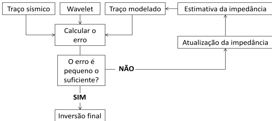
Figura 21: Fluxograma para a técnica de inversão determinística model-based
