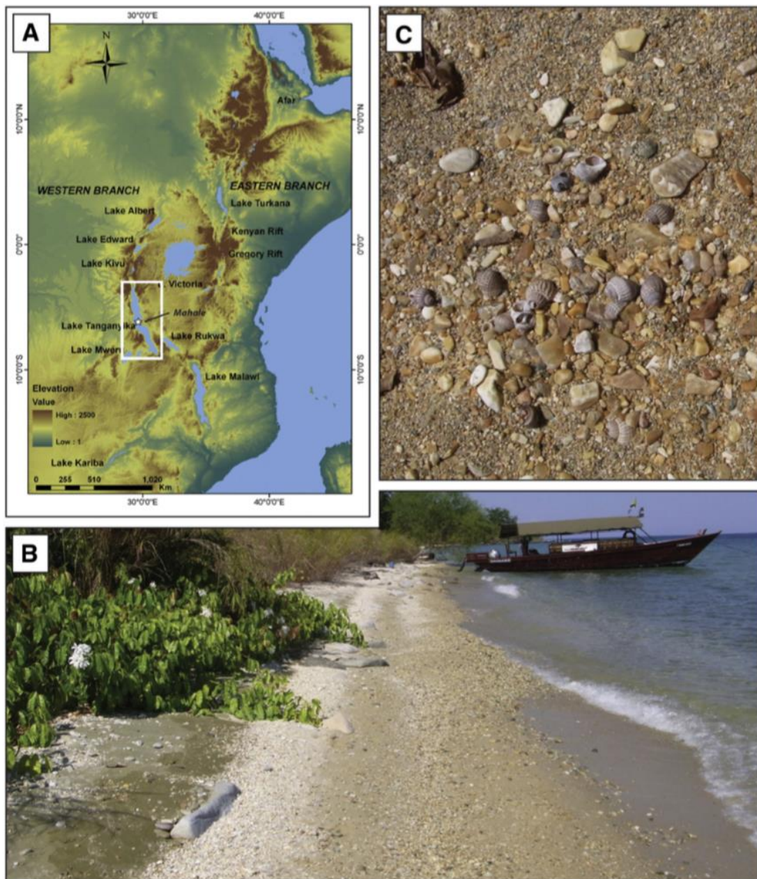
Figura 12: (A) Mapa de elevação do Sistema de Riftes do Leste Africano. (B) Formação de coquinas de coquinas ao longo da resgião costeira; (C) Coquina de gastrópodes em formação (Thompson et al. , 2015).
