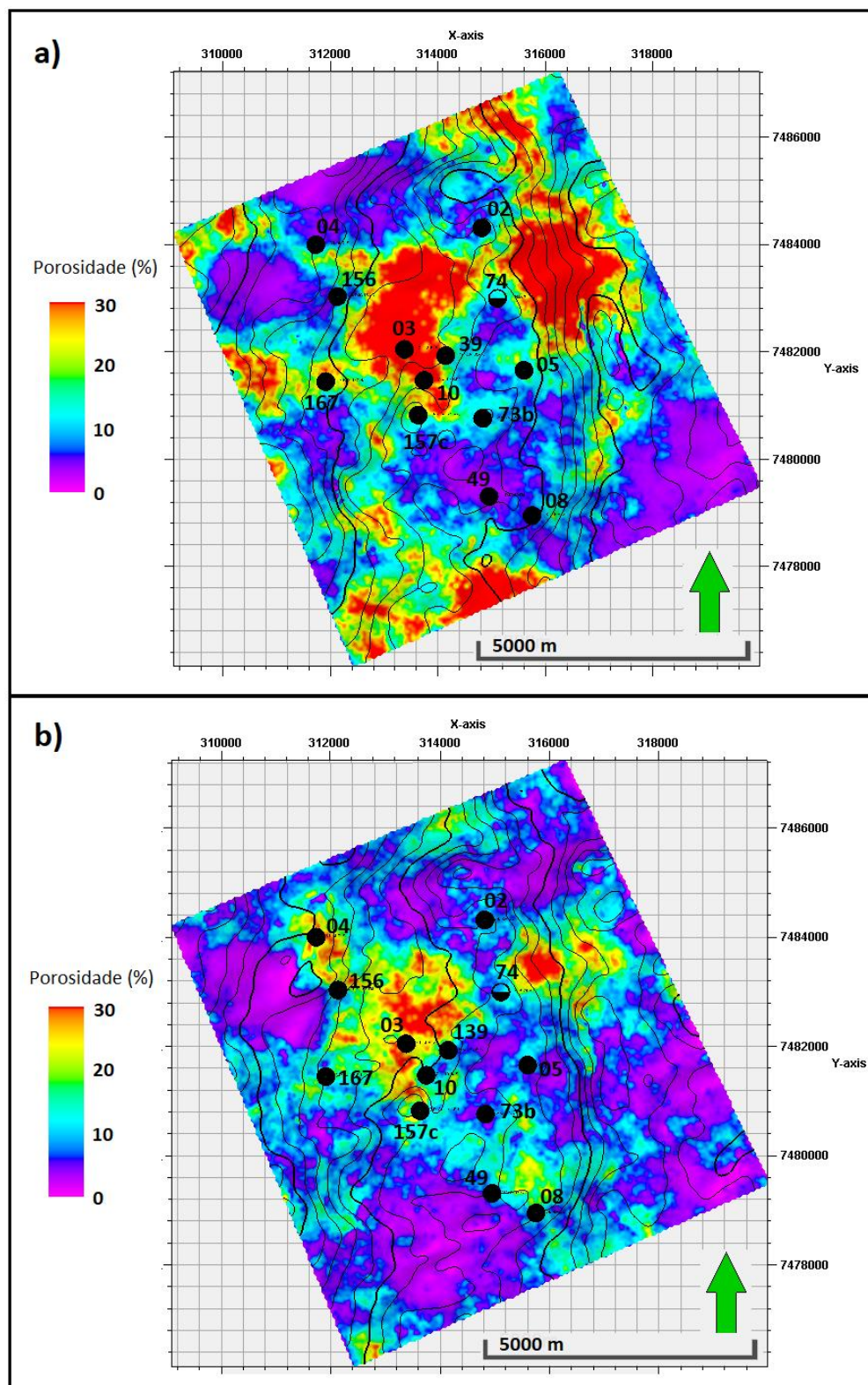
Figura 51: Mapas de porosidade dos níveis de coquina inferior (a) e coquina superior (b).
