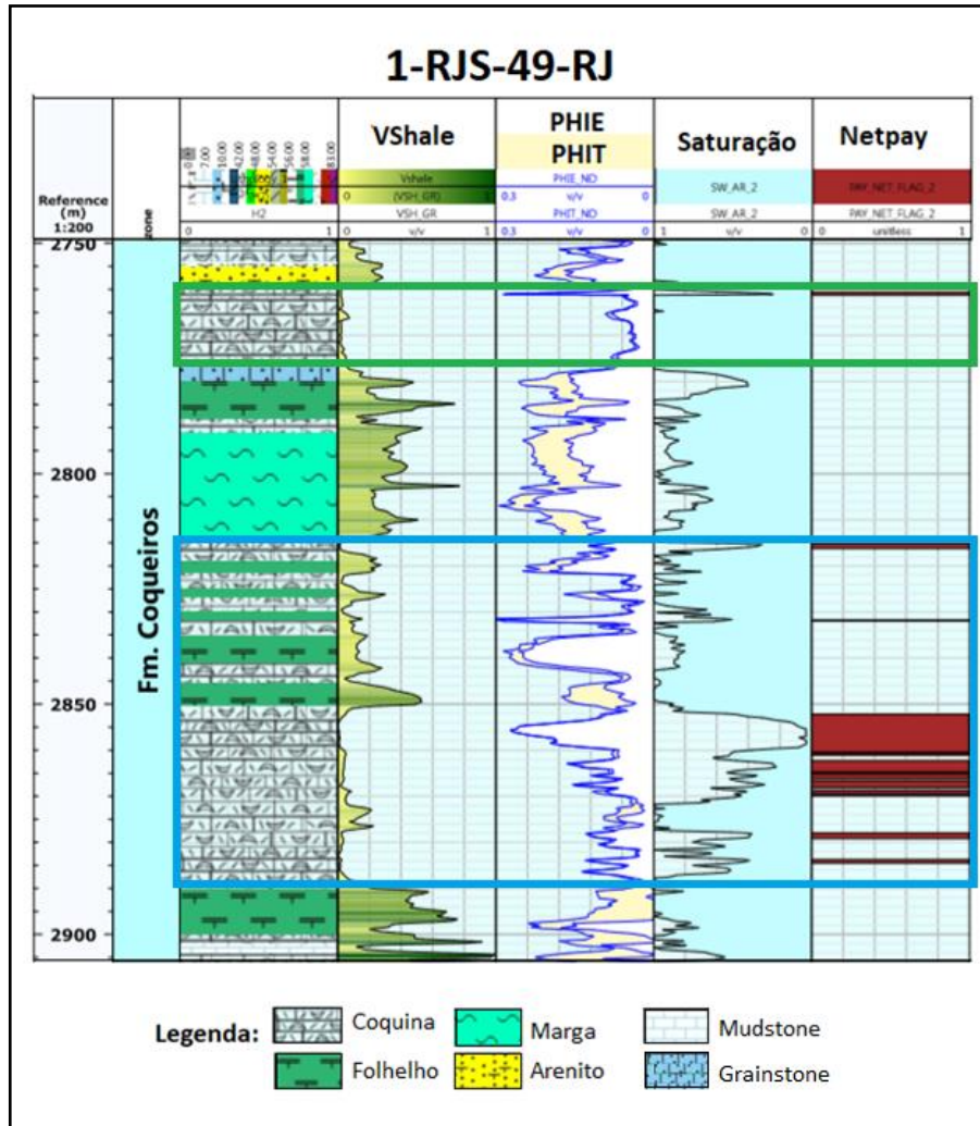
Figura 46: Resultado da análise petrofísica no poço 1-RJS-49-RJ. Track 1: Formação Coqueiros; track 2 fácies interpretadas; track 3: volume de argila (VShale); track 4: porosidade total (PHIT) e porosidade efetiva (PHIE); track 5: saturação de água; track 6: net-pay , Coquina superior: retângulo verde, coquina inferior: retângulo azul.
