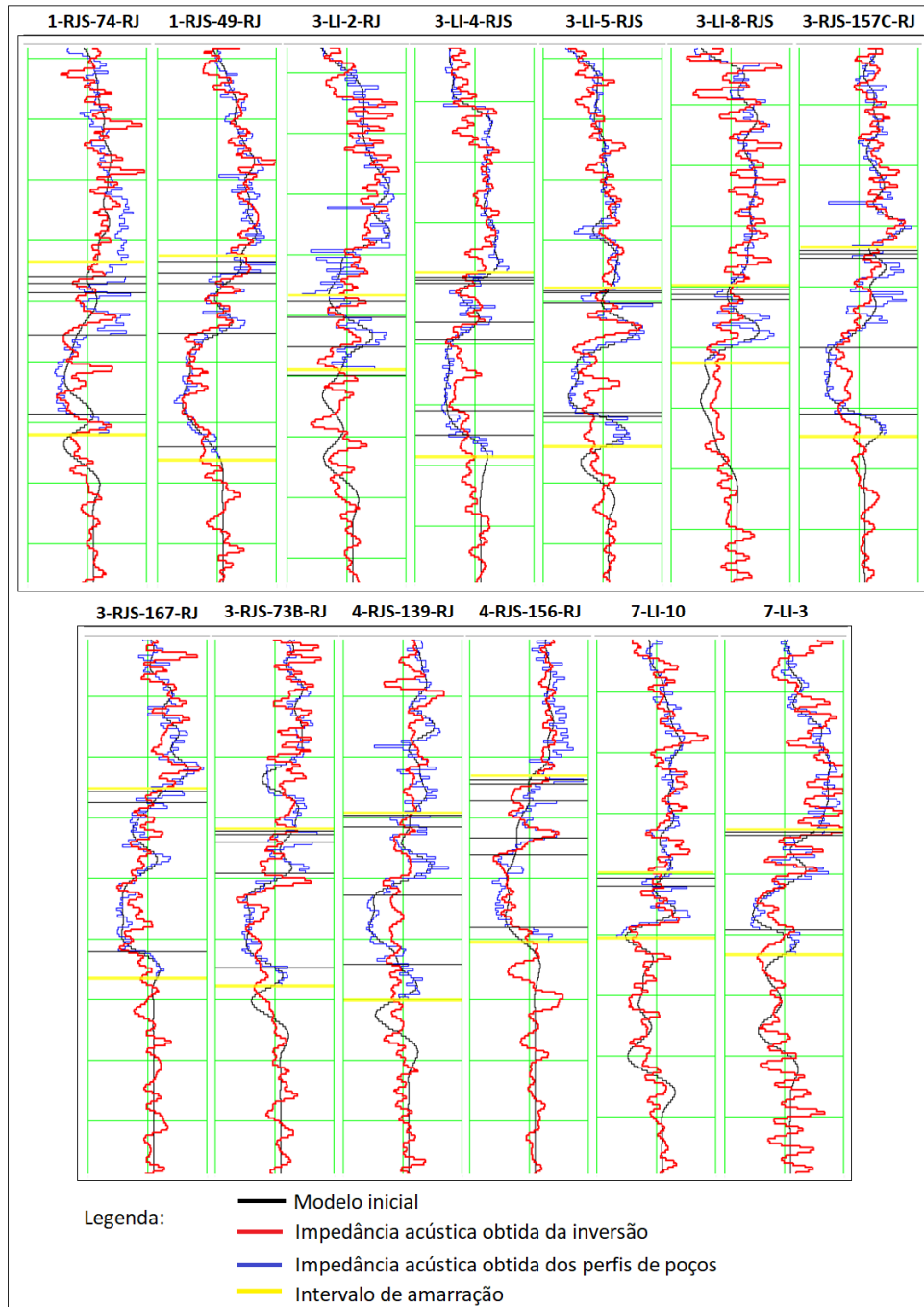
Figura 38: Resultados da inversão sísmica em cada um dos poços: impedância acústica obtida dos perfis de poços (curva azul), impedância acústica obtida da inversão (curva vermelha) e modelo de inicial de baixa frequência (curva preta).
