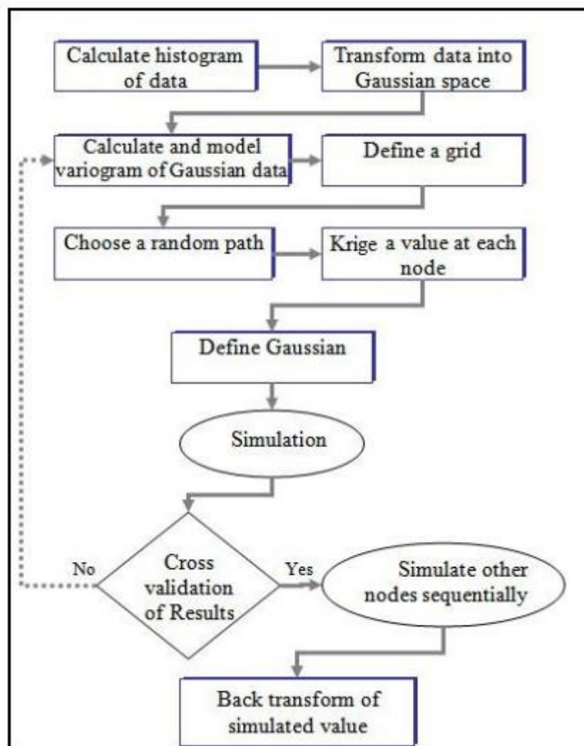
Figura 26: Etapas básicas do algoritmo de Simulação Sequencial Gaussiana (Deustch & Journel, 1992).
