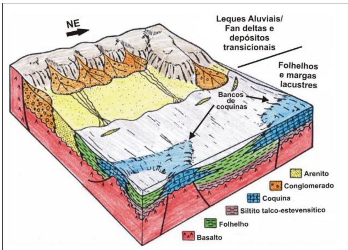
Figura 8: Modelo deposicional dos carbonatos lacustres do Grupo Lagoa Feia. Os bancos de coquinas se concentram no topo dos altos sindeposicionais do embasamento. Fonte: Adaptado de Guardado et al. , 1989.
