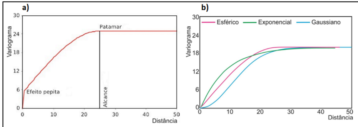
Figura 24: Propriedades do variograma (a) e tipos de modelos teóricos de variogramas (b). Fonte: Modificado de Yamamoto & Landim, 2013.
