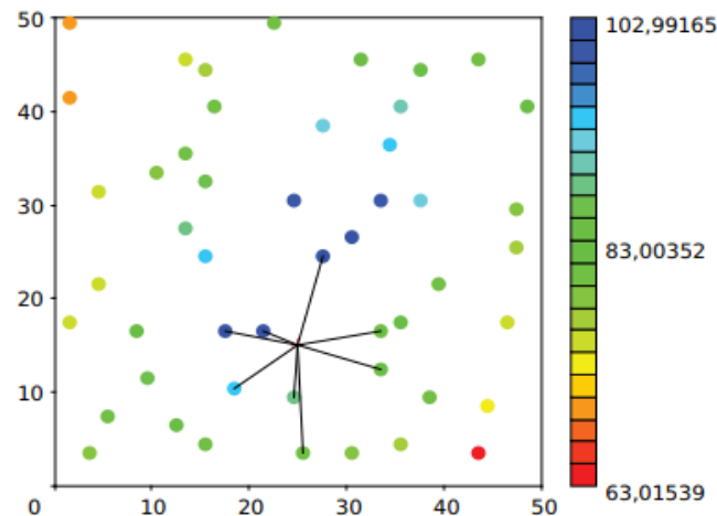
Figura 25: Exemplo de estimativa de um ponto não amostrado, a partir da combinação linear das amostras próximas de uma variável qualquer. Fonte: Yamamoto e Landim, 2013
