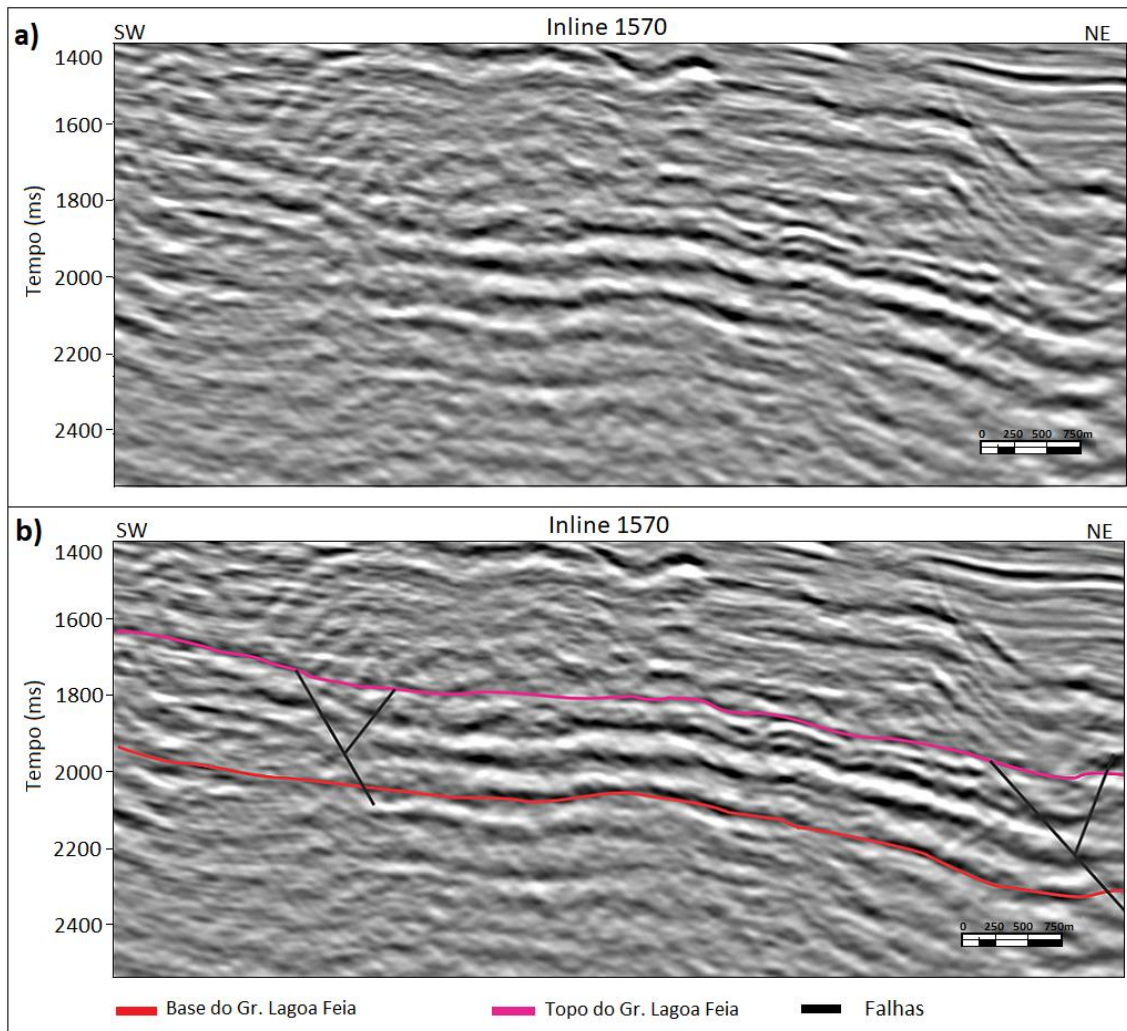
Figura 35: (a) Seção sísmica, inline 1570, sem interpretação; (b) seção sísmica, inline 1570, mostrando as discordância Topo Basalto (base do Grupo Lagoa Feia) e a discordância pré-Evaporítica (topo do Grupo Lagoa Feia) e as falhas no intervalo de interesse.
