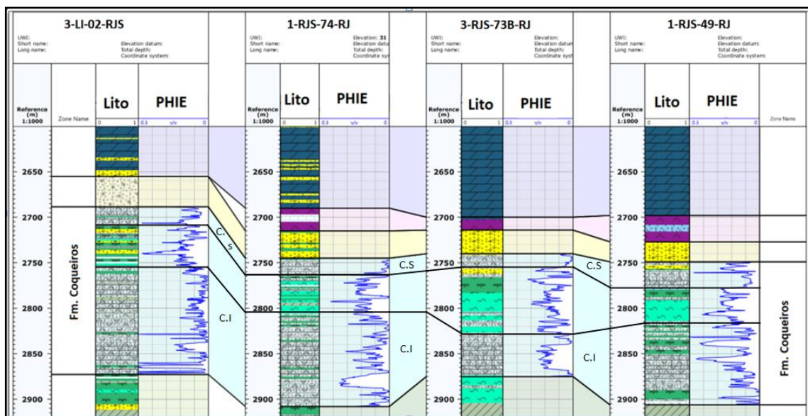
Figura 48: Correlação dos poços 3-LI-2-RJS, 1-RJS-74-RJ, 3-RJS-73B-RJ e 1-RJS-49-RJ com destaque a Formação Coqueiros. C.I: coquina inferior, C.S: coquina superior.
