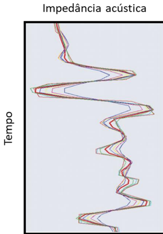
Figura 22: Ilustração da convergência dos modelos de impedância com sucessivas perturbações do algoritmo GLI . Em azul o modelo de impedância inicial fornecido pelo usuário e sucessivas iterações convergindo na solução final, em vermelho. (COOKE & CANT, 2010)
