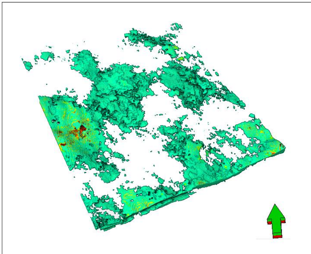
Figura 53: Geobody construído a partir do modelo de porosidade com cutoff de 13 a 30% de porosidade .
