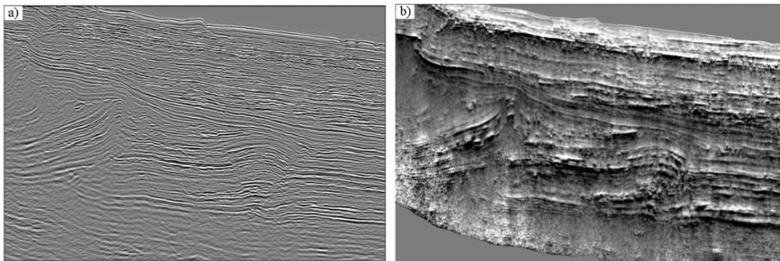
Figura 16: a) seção sísmica convencional e b) seção sísmica de a) aplicada a tecVA com rotação de fase. (Bulhões e Amorim, 2005, fornecido pela CGG).
