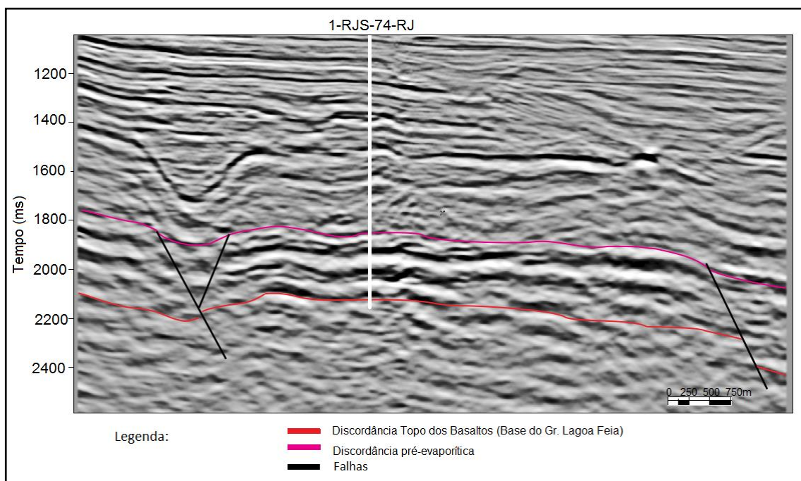
Figura 39: Seção sísmica original na crossline 1438 com o poço 1-RJS-74-RJ.
