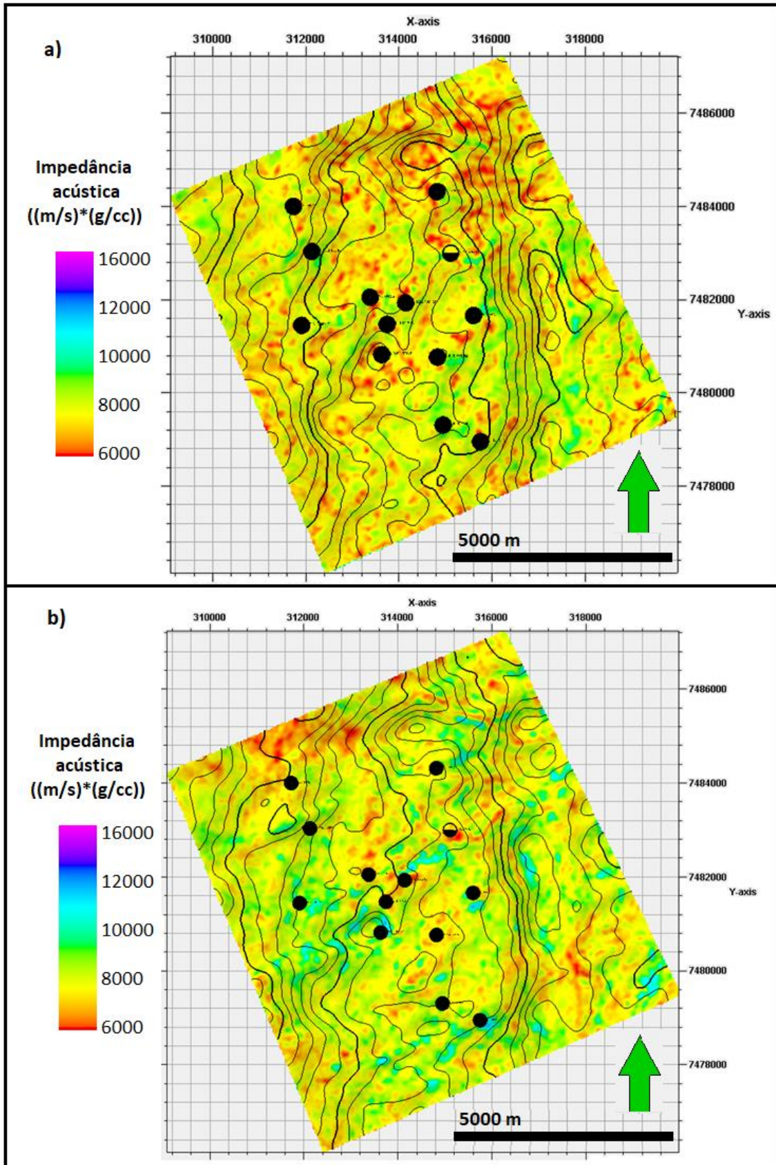
Figura 43: Mapas com os valores de impedância acústica sobre os topos das superfícies correspondentes a cozinha inferior (a) e a cozinha superior (b).
