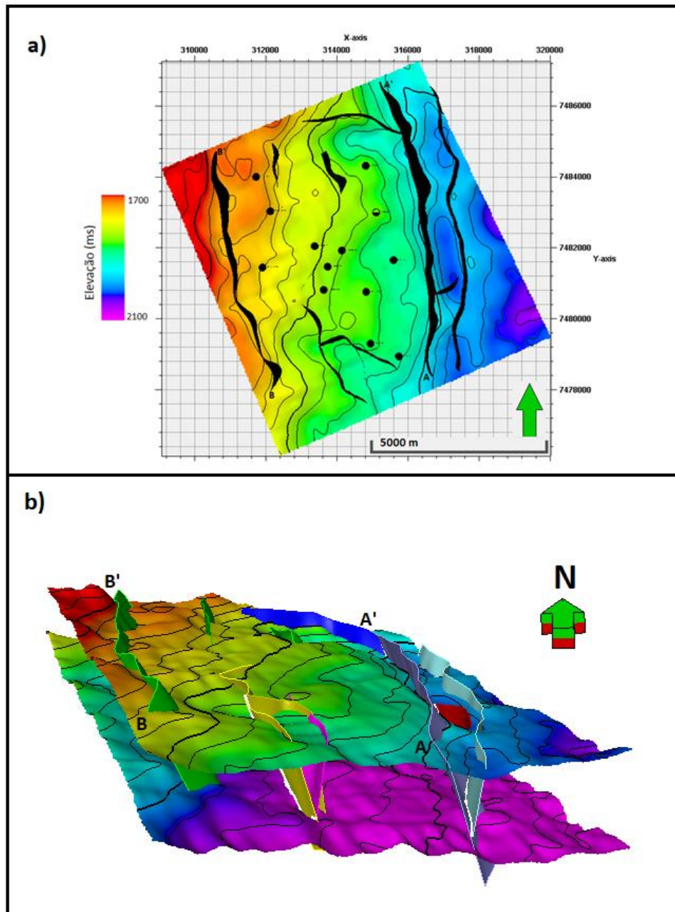
Figura 36: (a) Mapa de superfície da discordância pré-evaporítica (topo do Gr. Lagoa Feira) e (b) visão 3D dos horizontes topo e base do Gr. Lagoa Feia e falhas mapeadas que serviram de modelo estrutural para a inversão.
