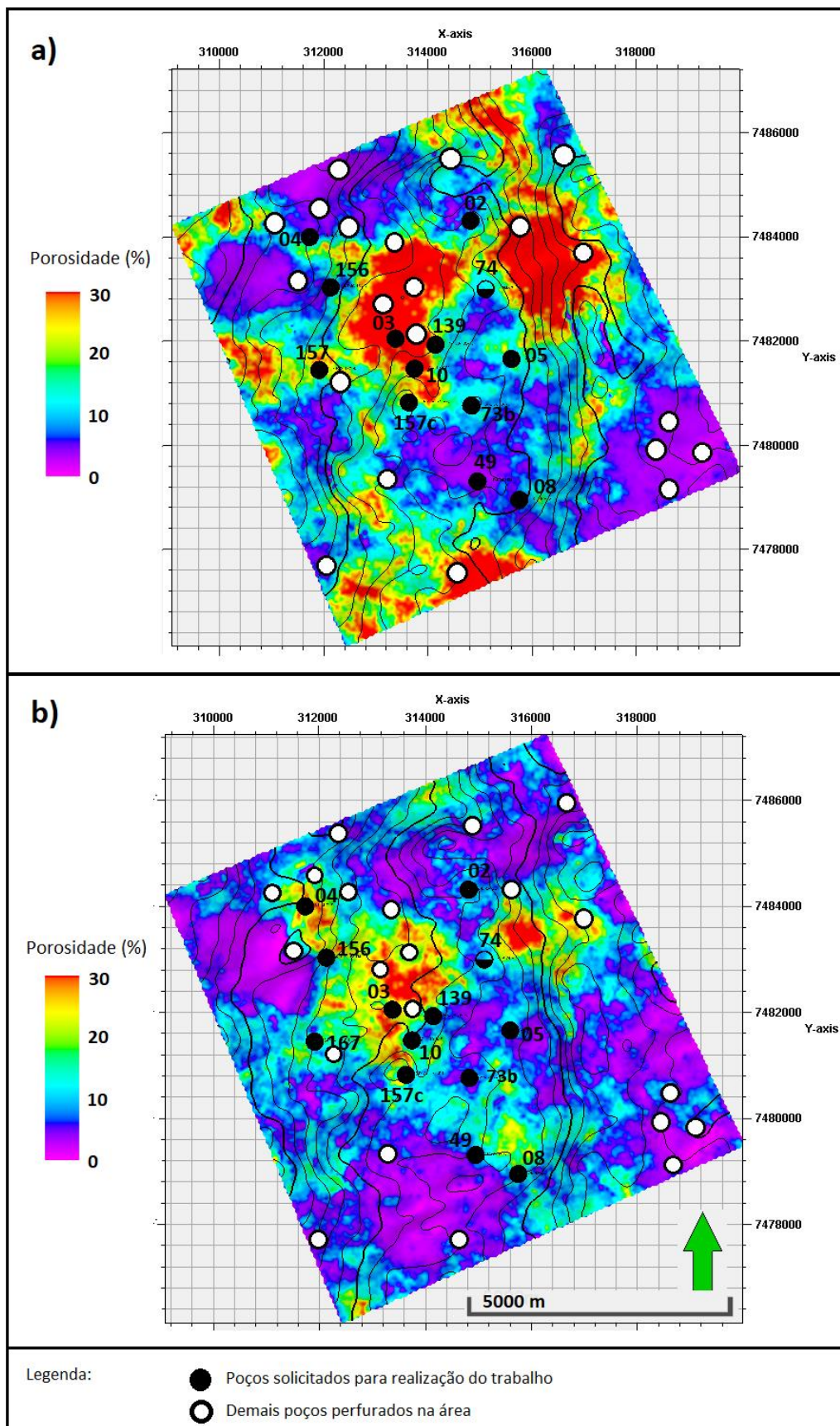
Figura 52: Mapas de porosidade da coquina inferior (a) e coquina superior (b).
