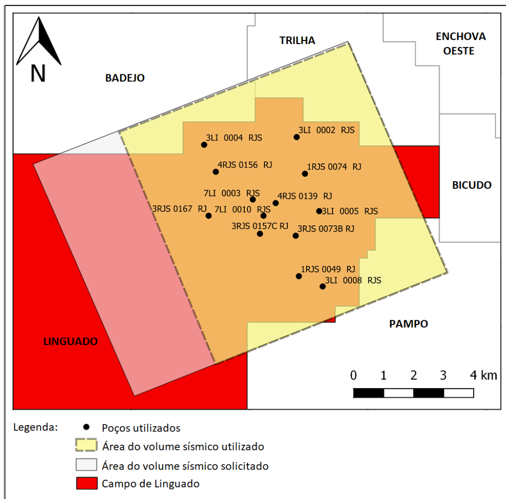
Figura 27: Mapa de localização dos dados utilizados no presente estudo.
