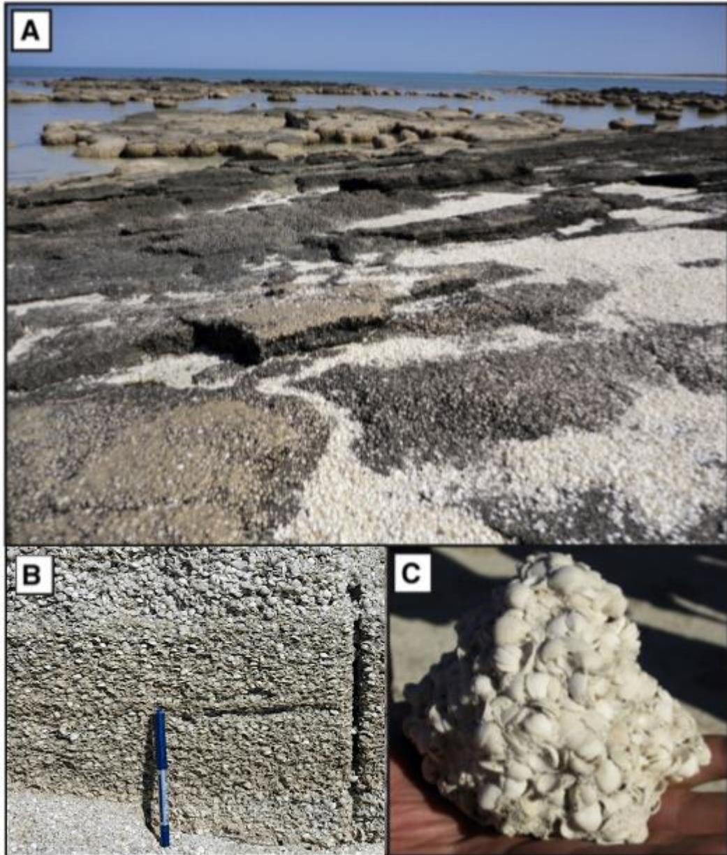
Figura 11: Camadas parcialmente litificadas de coquinas gradam em direção ao mar para estromatólitos dômicos (Thompson et al. , 2015); (B) Camadas parcialmente litificadas de coquinas (Fotografia de Marcelo Blauth em Bizotto, 2014); (C) Coquina de bivalves cimentada com matriz arenosa (S.F. Poropat, 2008 em Thompson et al. , 2015)
