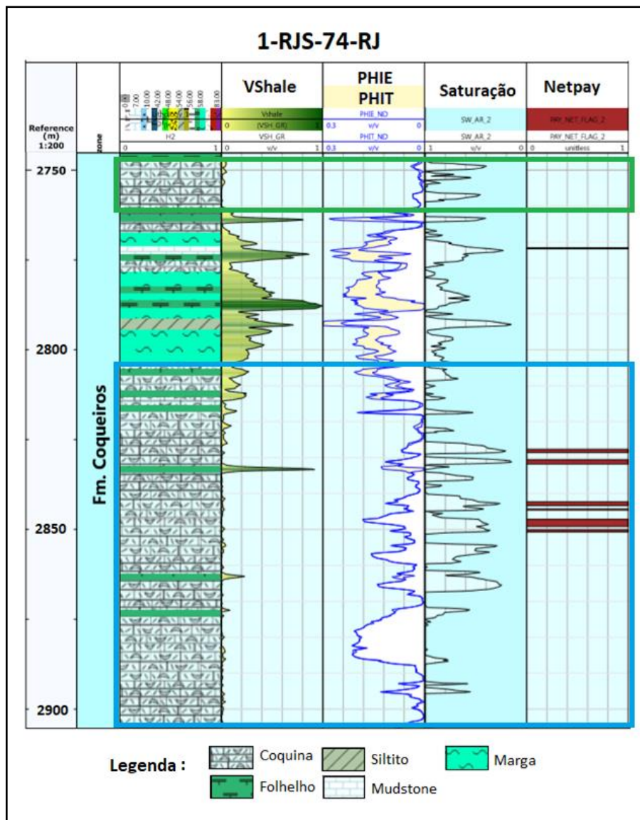
Figura 47: Resultado da análise petrofísica no poço 1-RJS-74. Track 1: Formação Coqueiros; track 2: fácies interpretadas; track 3: volume de argila (VShale); track 4: porosidade total (PHIT) e porosidade efetiva (PHIE); track 5: saturação de água; track 6: net-pay , Coquina superior: retângulo verde, coquina inferior: retângulo azul.
