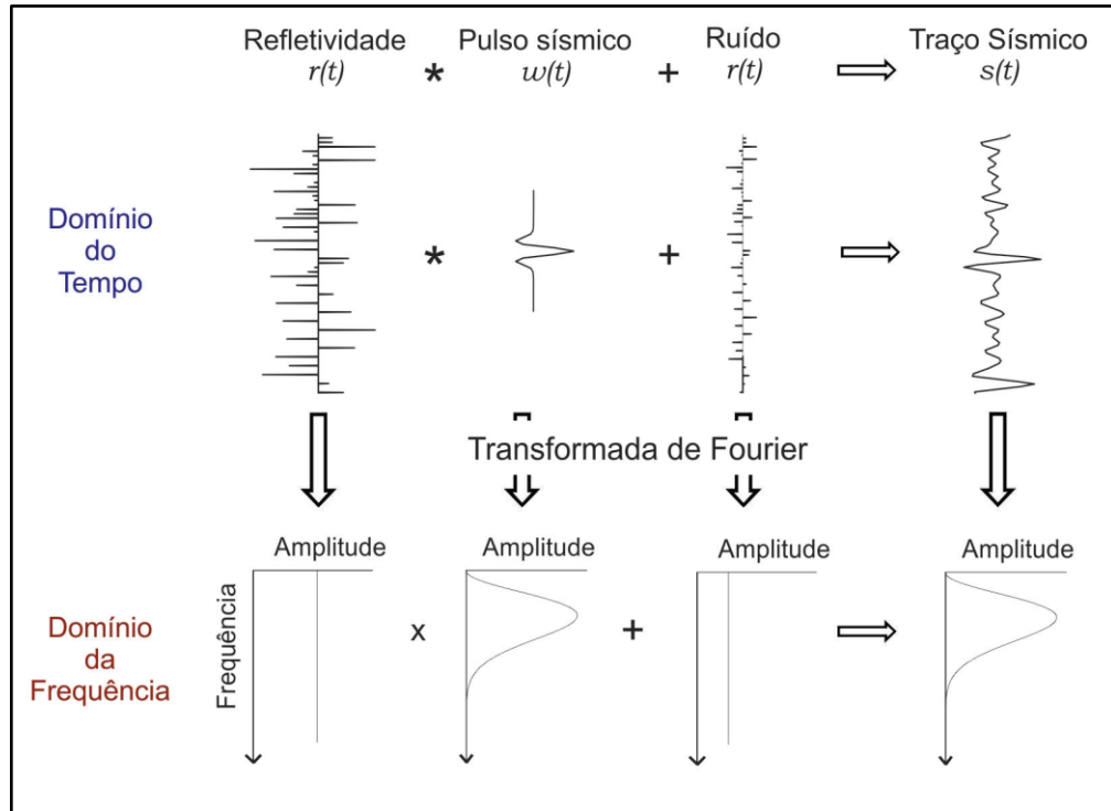
Figura 19: O modelo convolucional do traço sísmico e a transformada de Fourier da função refletividade, do pulso sísmico, do ruído e do traço sísmico (Lupinacci, 2014).
