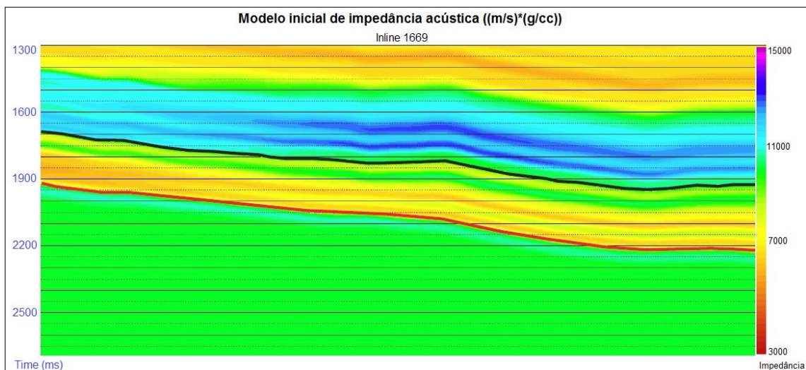
Figura 32: Modelo inicial de impedância acústica suavizado obtido a partir da interpolação dos dados de poços.
