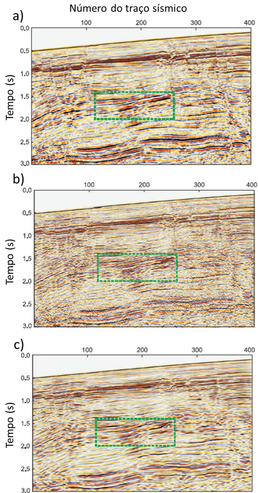
Figura 15:(a) seção sísmica original; (b) seção sísmica com aplicação da filtragem Q inversa mostrada; (c) seção sísmica com a aplicação da metodologia proposta por Lupinacci et al. (2017). Modificado a partir de Lupinacci et al. (2017).
