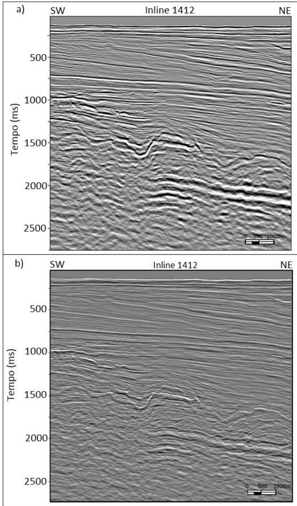
Figura 37: (a) Seção sísmica original, inline 1412; (b) sísmica pré-condicionada, inline 1412, usando a filtragem curvelet, filtro inverso Q e filtro passa banda em 60Hz.
