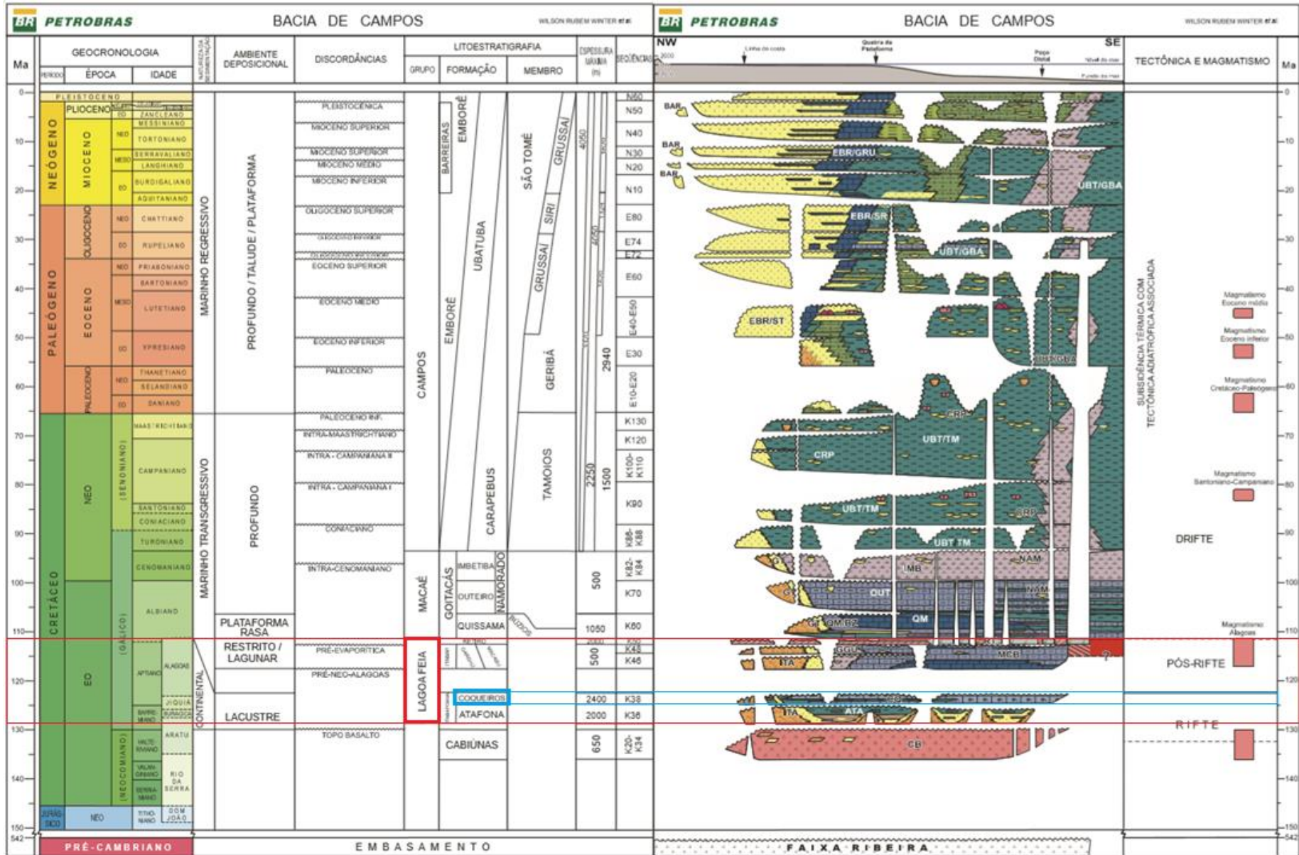
Figura 3: Carta cronoestratigráfica da Bacia de Campos com destaque para a Formação Coqueiros, alvo de estudo. Fonte: Winter et al., 2007
